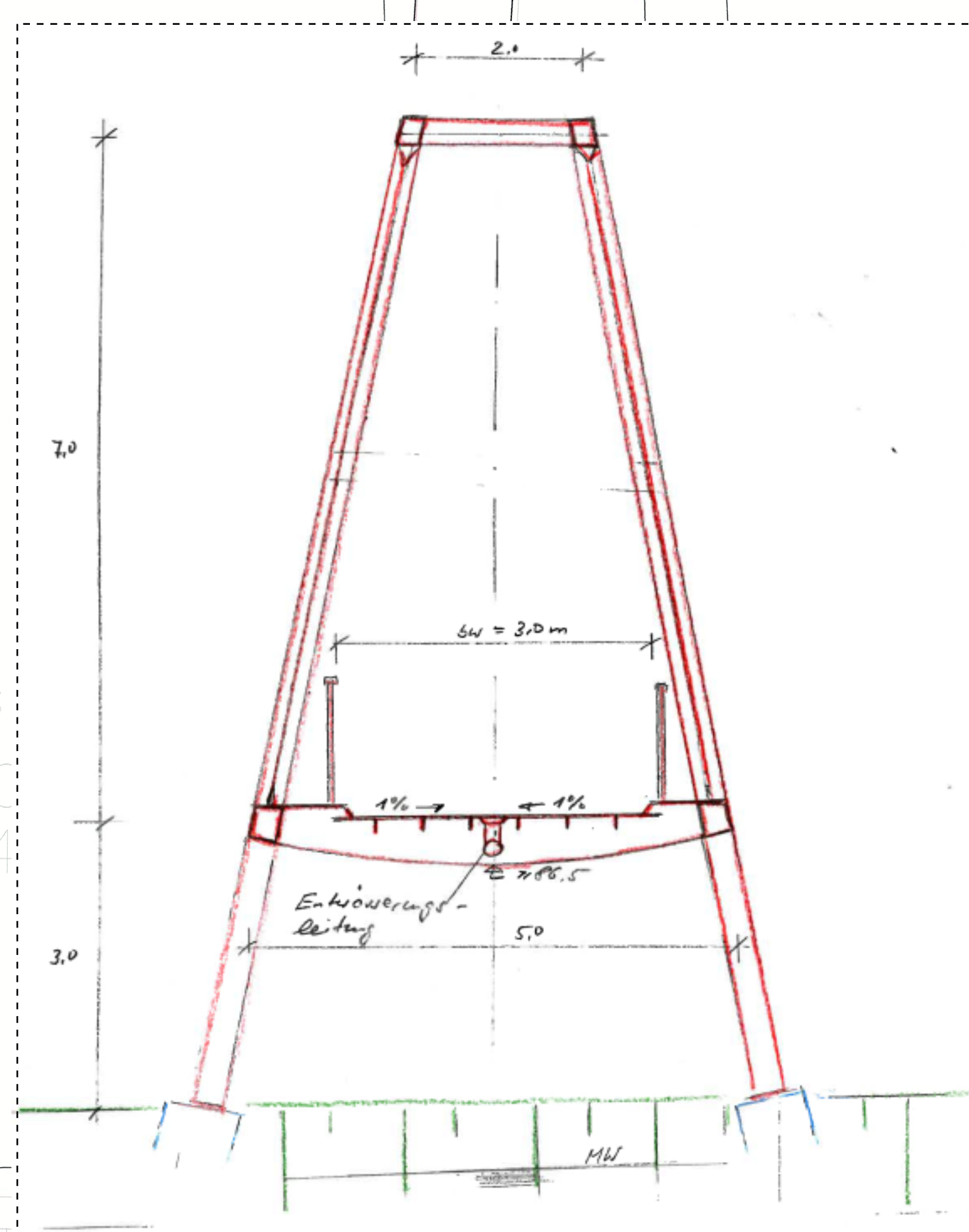
Querschnitt M1:50
