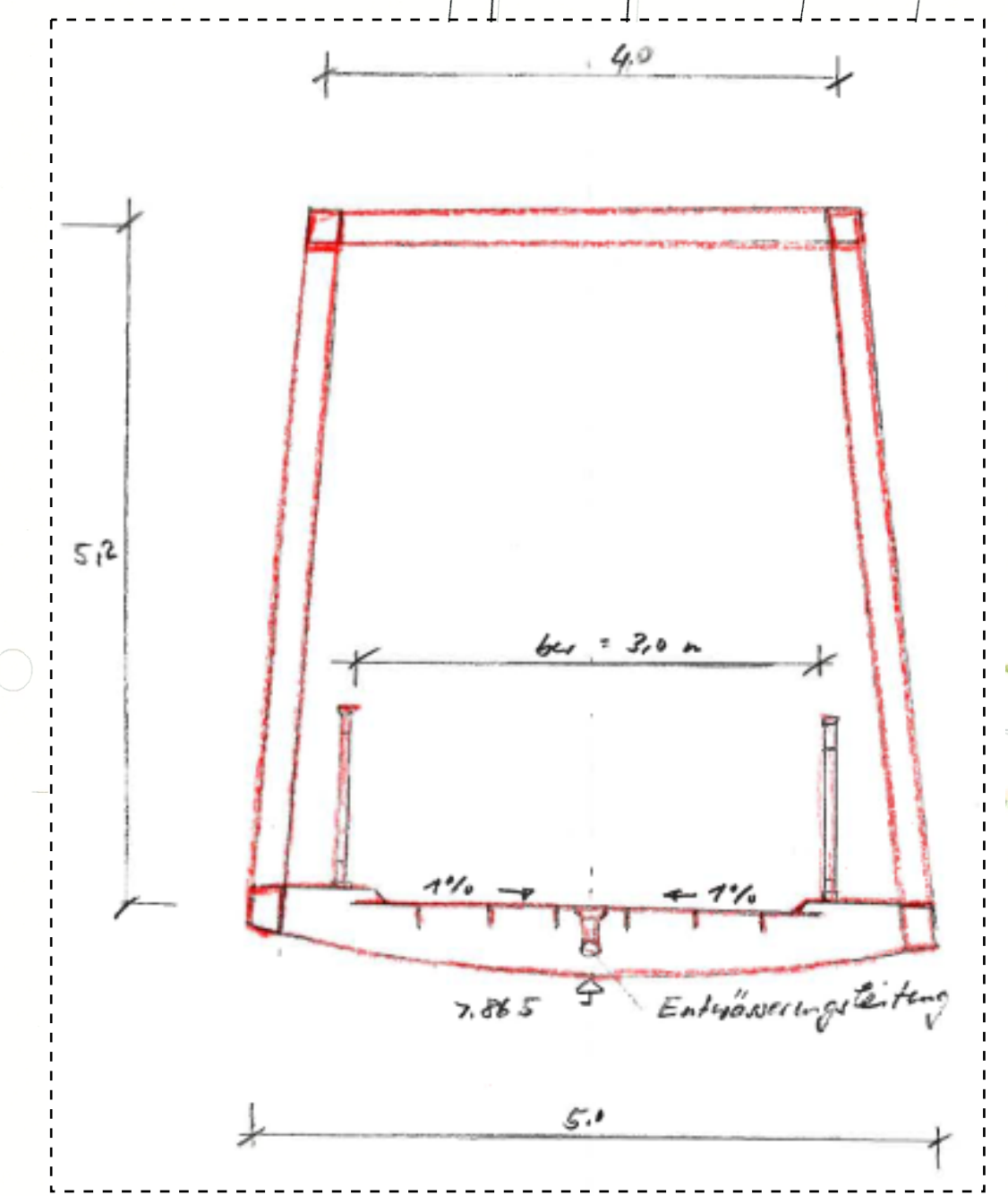
Querschnitt M1:50
