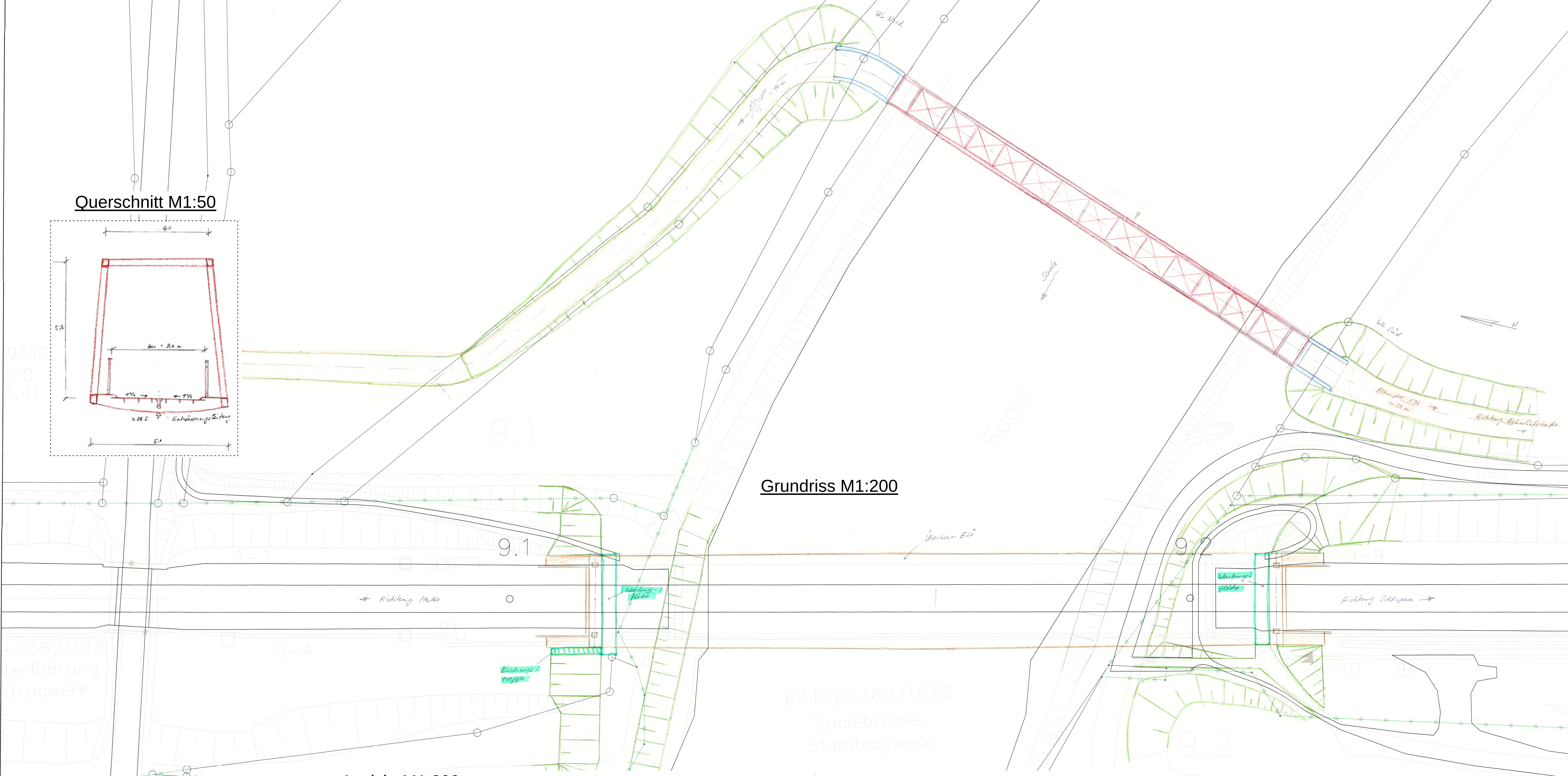
Ansicht M1:200
