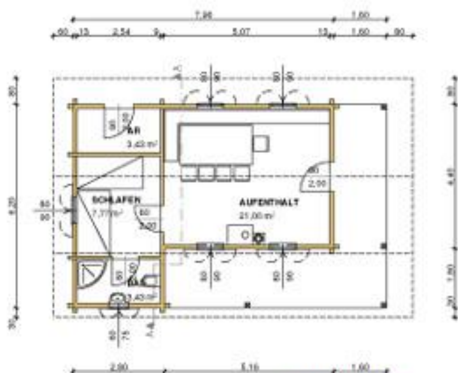
GRUNDRISS
